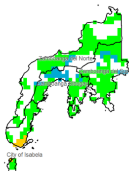
NDVI
