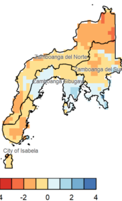
SPEI3 (Aug-Sep-Oct)
