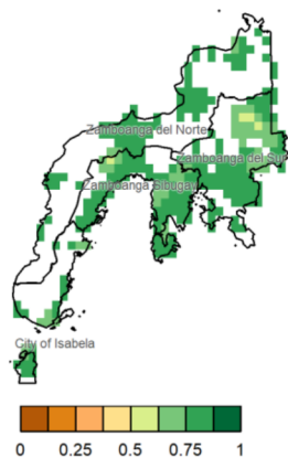
NDVI
